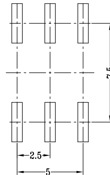
P.C.B LAYOUT
